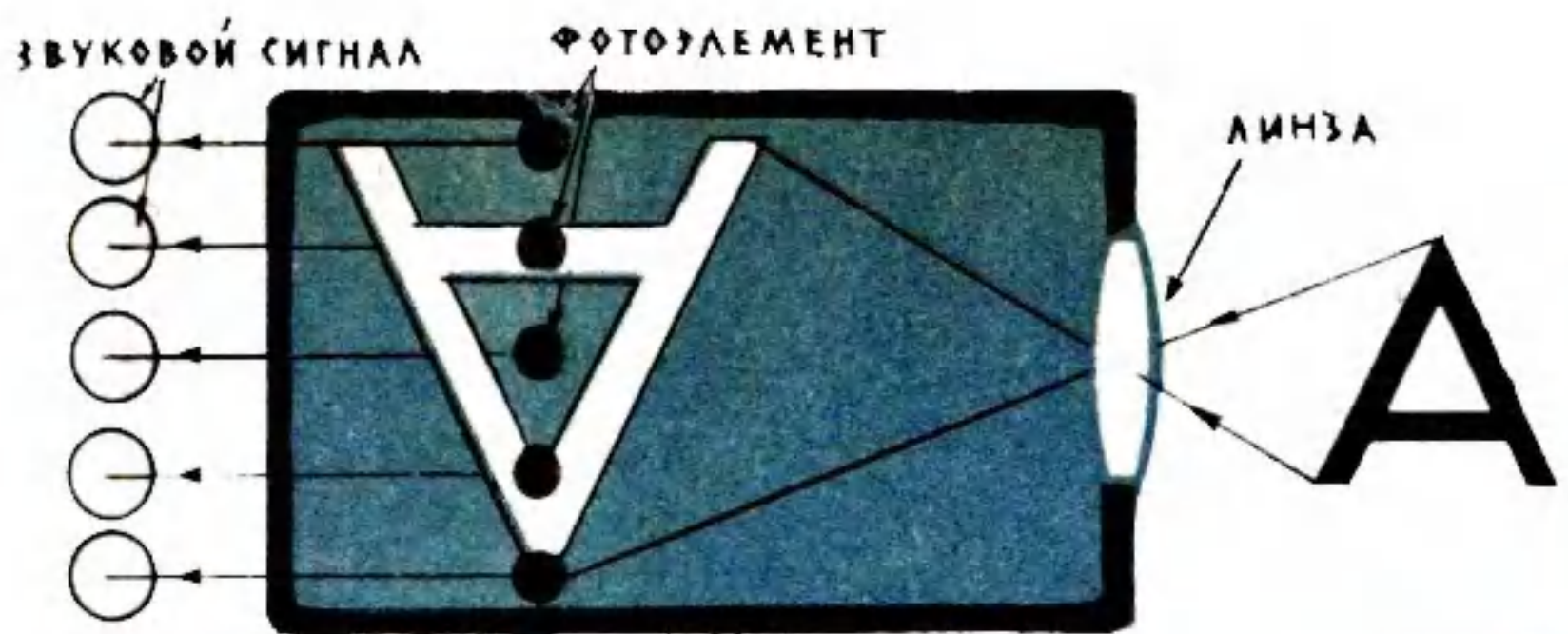
ПРИНЦИП УСТРОЙСТВА ТЮРИНА
